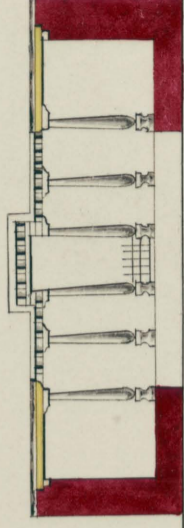
Планы и разрезъ Шайх-Нурдина Басира.
